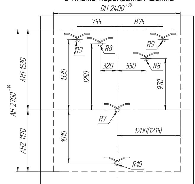
Схема расположения монтажных петель в плите перекрытия шахты
